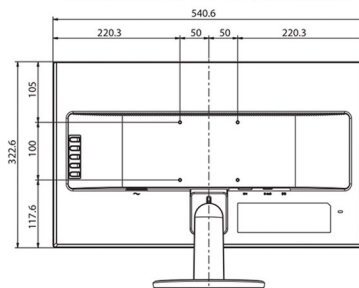
Dimensiones del Monitor
